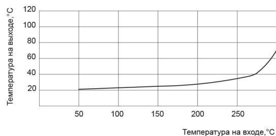
График для отвода-охладителя OC200-OX50
